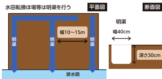
【図2】明渠づくり概略(一例)
